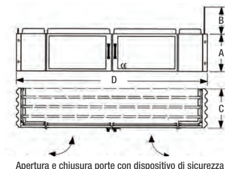
Apertura e chiusura porte con dispositivo di sicurezza
